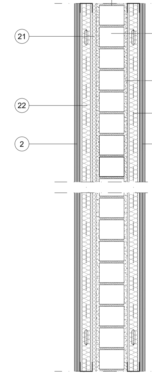
T10 Tabique múltiple compuesto por fábrica de ladrillo cerámico perforado de 11.5 cm de espesor + trasdosado doble placa normal sobre subestructura de 48 mm con lana de roca de 40 mm y 70 Kg/m 3 + trasdosado doble placa normal sobre subestructura de 48 mm con lana de roca de 40 mm y 70 Kg/m 3 . Incluida lámina de chovACUSTIC 35 fieltex o equivalente entre ladrillo panel y trasdosado en la cara del distribuidor.
