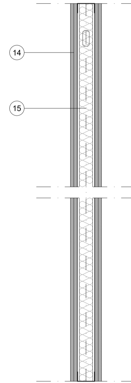
TF2 Falseado 48 mm + doble placa hidrofugada de 12.5 mm de espesor. Aislamiento acústico de lana mineral natural (LMN), no revestido, de 50 mm de espesor, resistencia térmica 1,15 m 2 K/W. Espesor total 140 mm. Aislamiento acústico a ruido aéreo 51.9 dBA. Resistencia al fuego EI-60.
