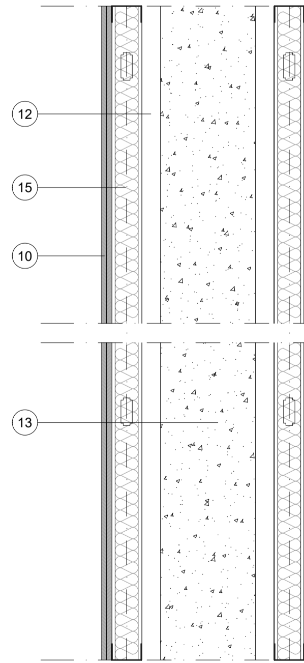
TF1 Falseado 48 mm + doble placa normal de 12.5 mm de espesor alta dureza. Aislamiento acústico de lana mineral natural (LMN), no revestido, de 50 mm de espesor, resistencia térmica 1,15 m 2 K/W. Espesor total 140 mm. Aislamiento acústico a ruido aéreo 51.9 dBA. Resistencia al fuego EI-60.
