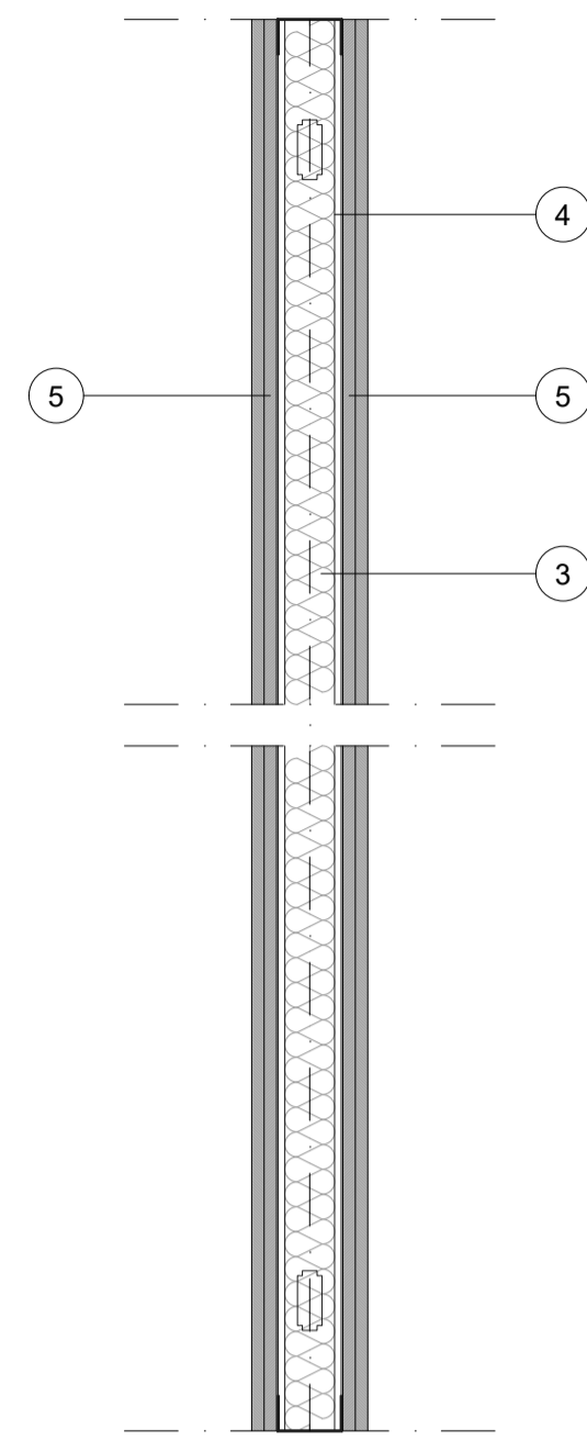
T3 PYL db hidrofugado de 90 mm + 2 placas de 15 mm hidrofugadas a cada lado. Tabique múltiple autoportante; aislamiento acústico de lana mineral natural (LMN), no revestido, de 60 mm de espesor, resistencia térmica 1,6 m 2 K/W. Espesor total 140 mm. Aislamiento acústico a ruido aéreo 51.9 dBA. Resistencia al fuego EI-60.
